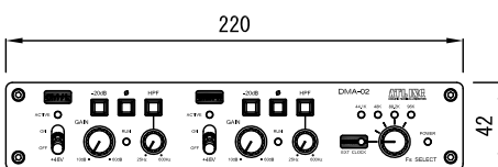
正面図
