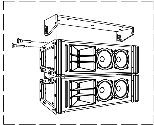
MUB-1D全体姿図
