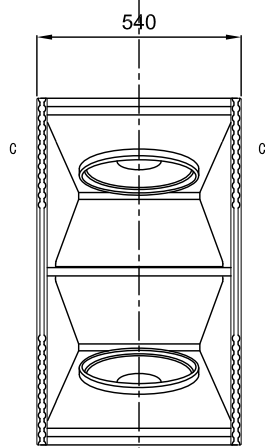
正面図
