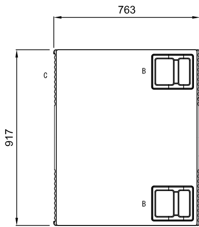
右側面図
