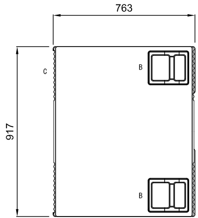
右側面図
