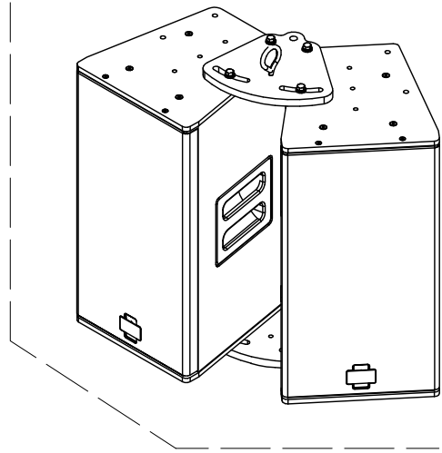
UPJにプレートを付けた姿図
