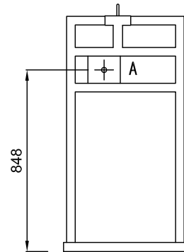
右側面図
