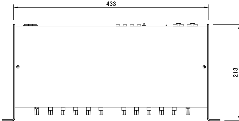
上面図
