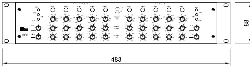
正面図
