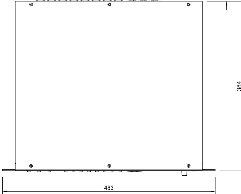
上面図
