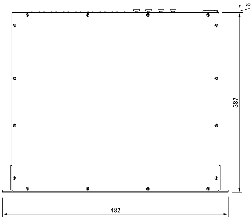
上面図
