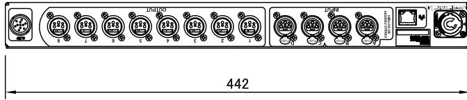
背面図
