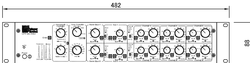
正面図
