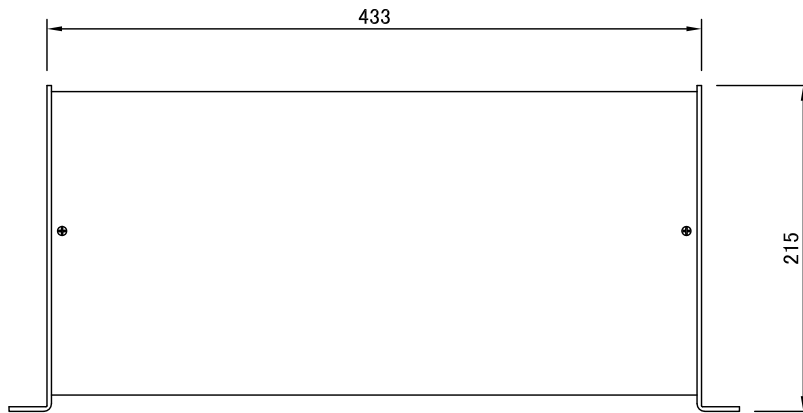
上面図
