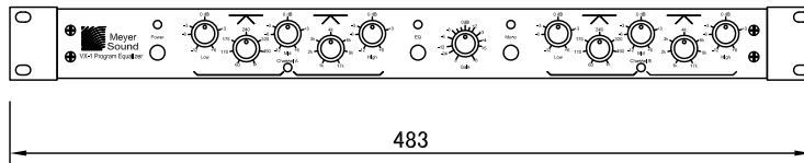
正面図
