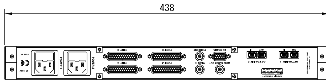
後面図
