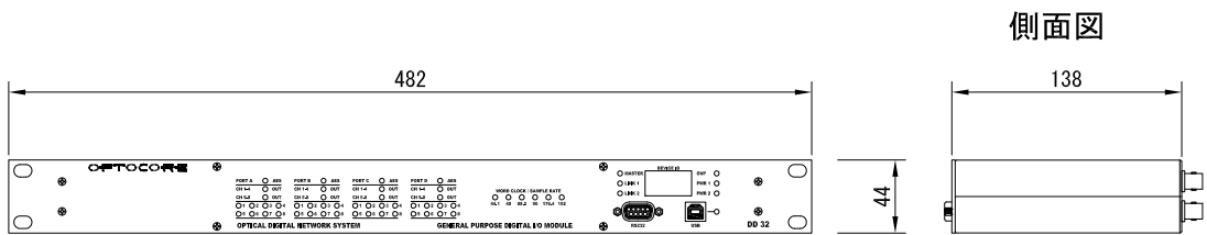
正面図
