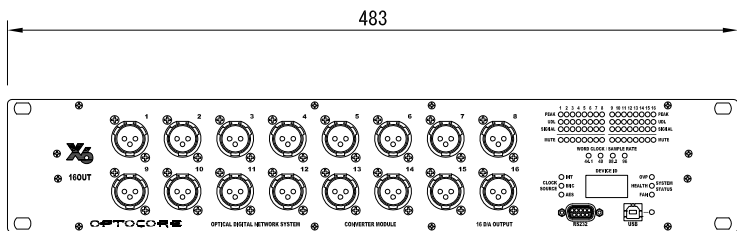
上面図
