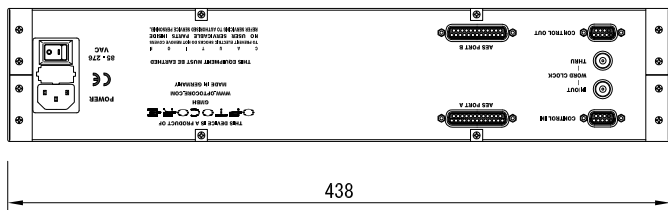
後面図
